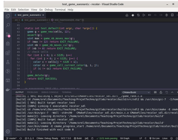
Environnement de programmation VSCode.
